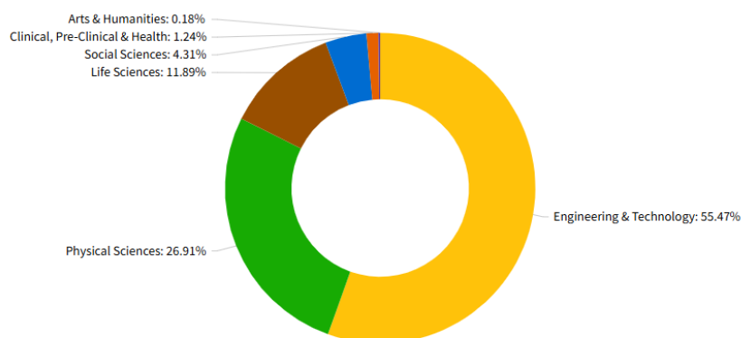
图 3 GIPP 学科分类论文占比
