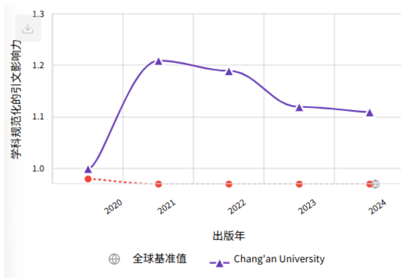
图 5 学科规范化的引文影响力
